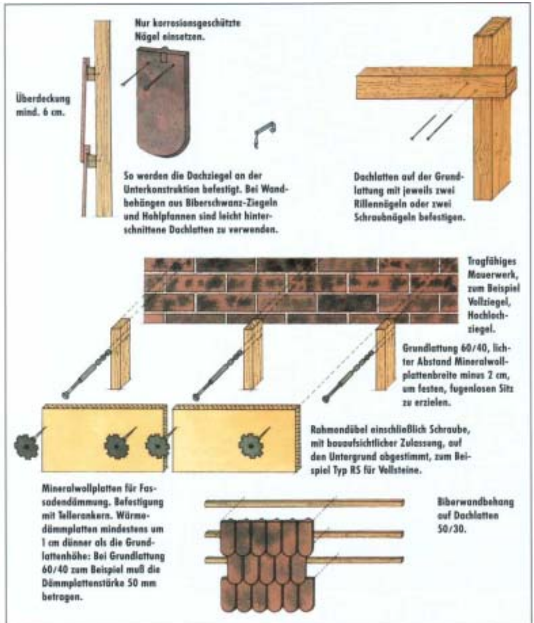
Den Fassadenteilen Schutz zu bieten, die dem Wetter besonders ausgesetzt waren, ist häufig der wichtigste Grund für einen Wandbehang aus Dachziegeln.
